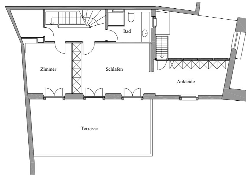
Obergeschoss
