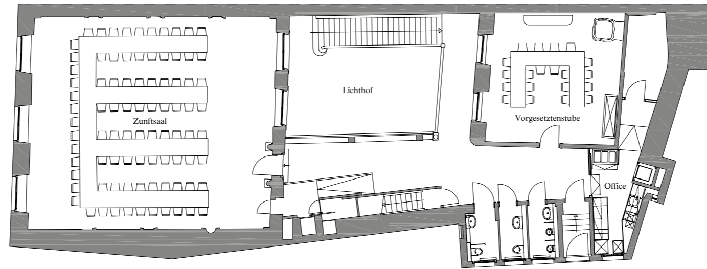
Grundriss Obergeschoss
